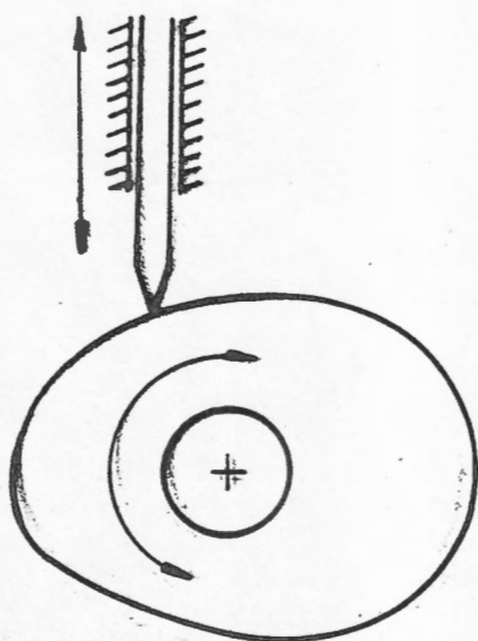
Seguidor puntual desplazado
