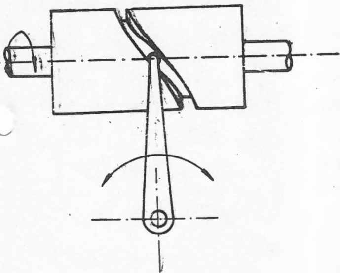
Leva cilíndrica
