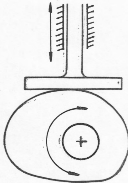
Seguidor plano
