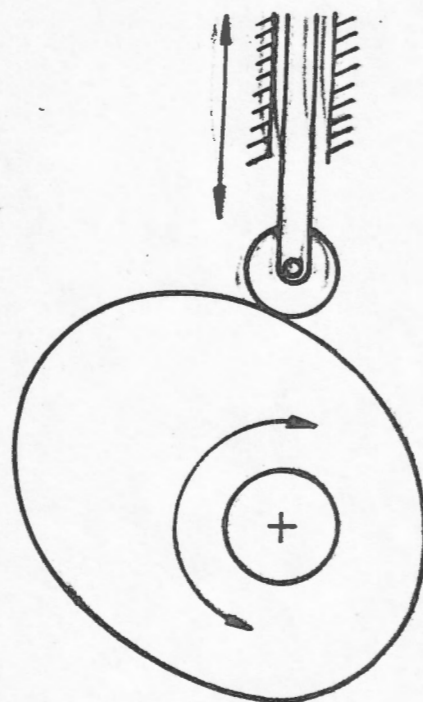
Seguidor de rodillos
