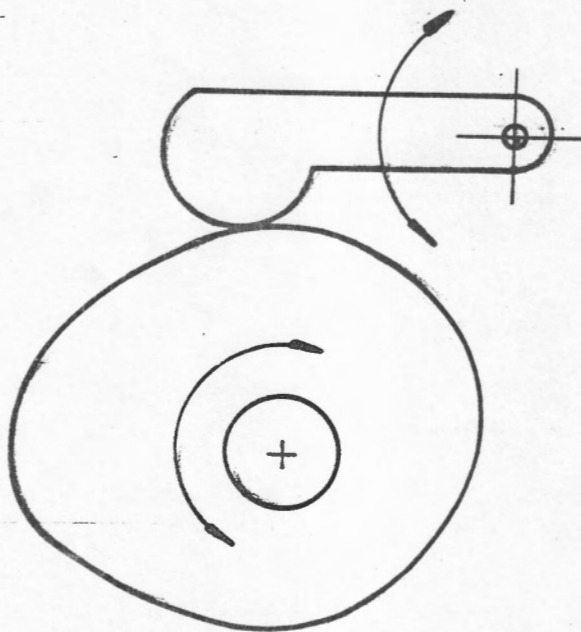
Seguidor oscilante
